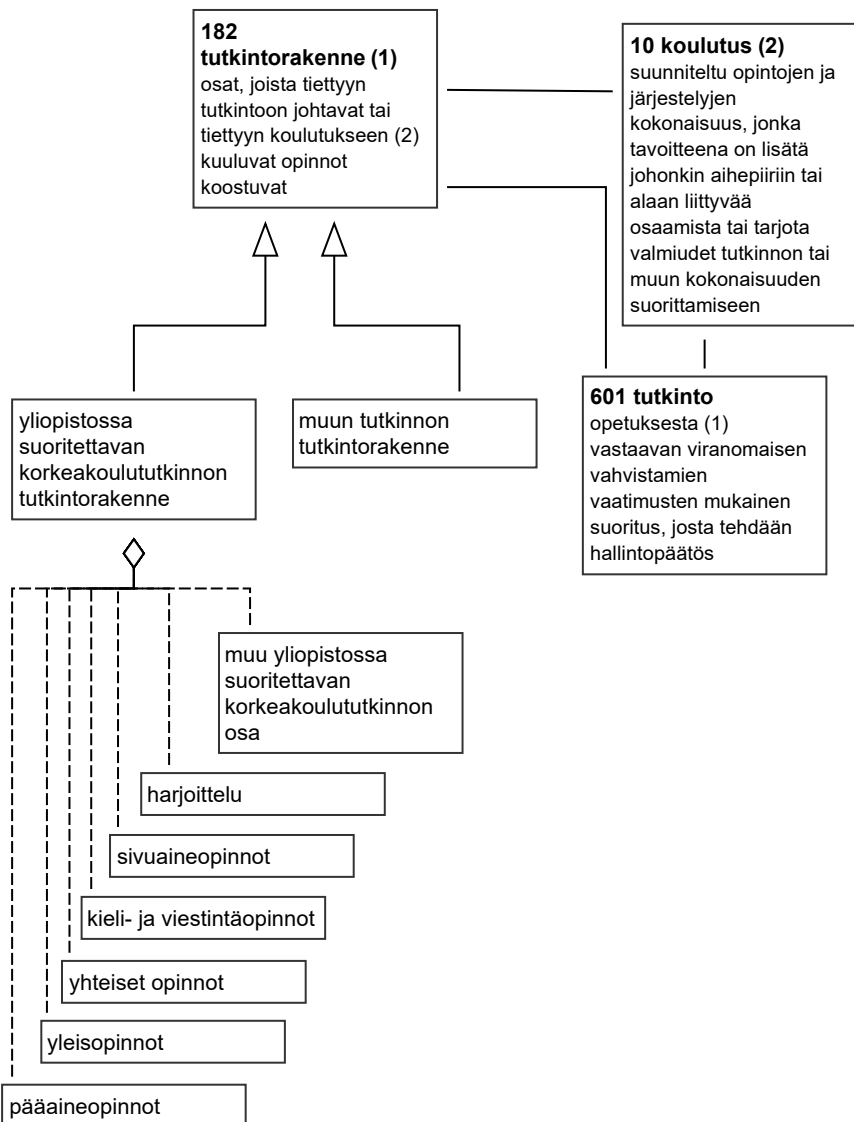
Käsitekaavio 21. Tutkintorakenne.
