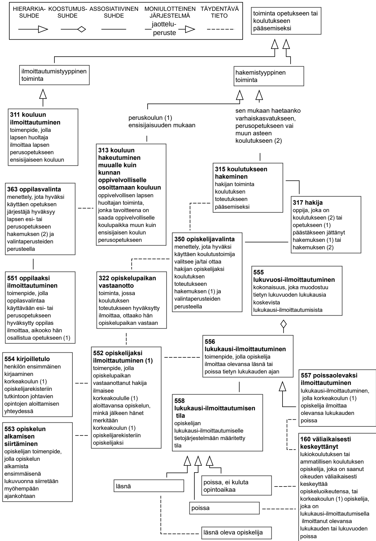
Käsittekaavio 62. Ilmoittautumiskäsitteitä.
