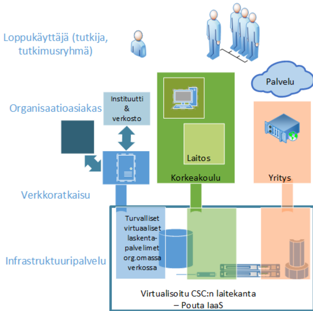
Kuva 9. IaaS-pilvipalvelumalli organisaatioille.
