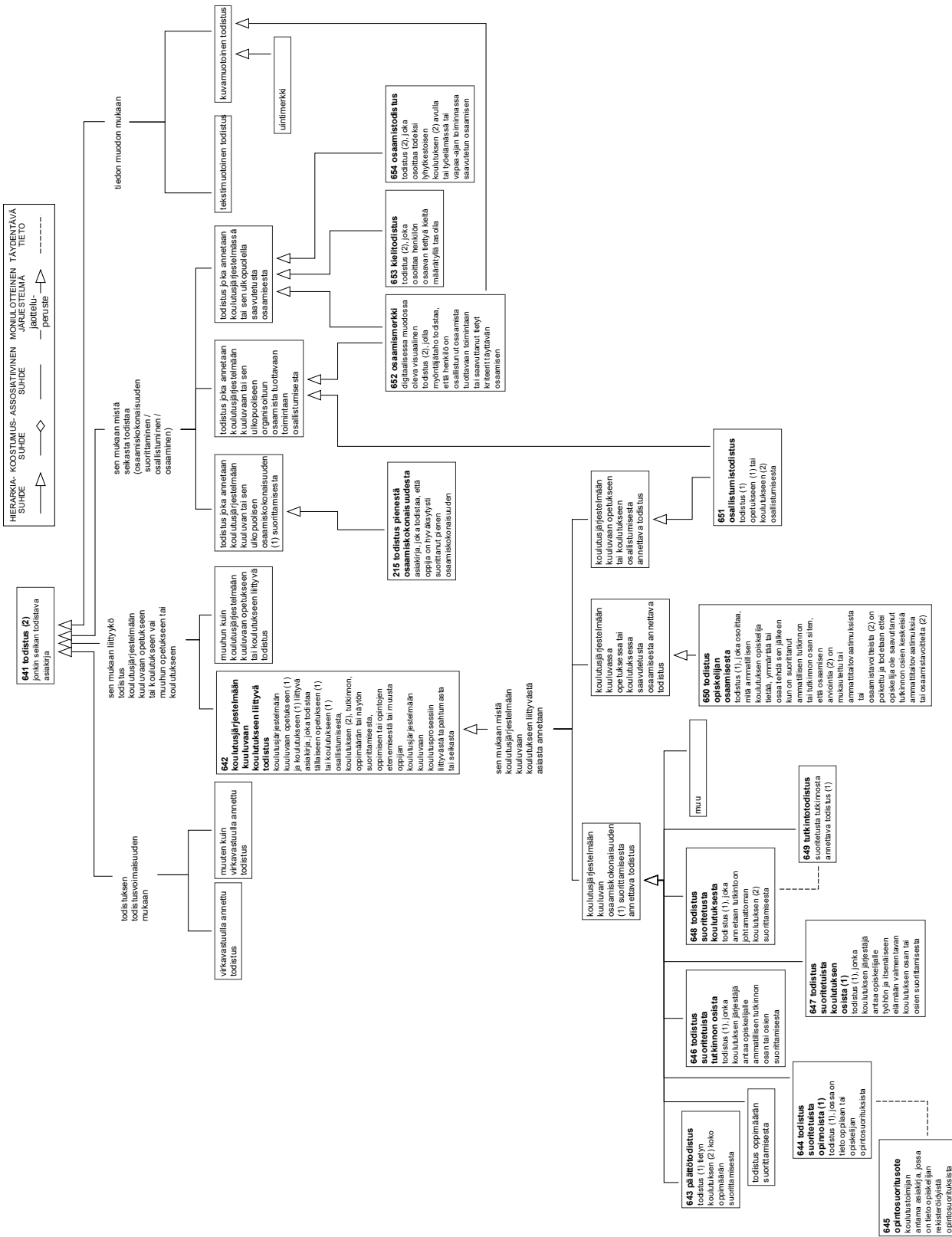
Käsittekaavio 75. Todistus.
