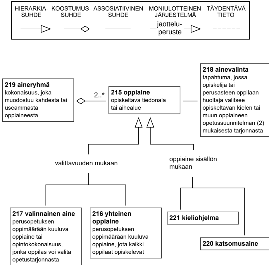
Käsitekaavio 28. Oppiaine.
