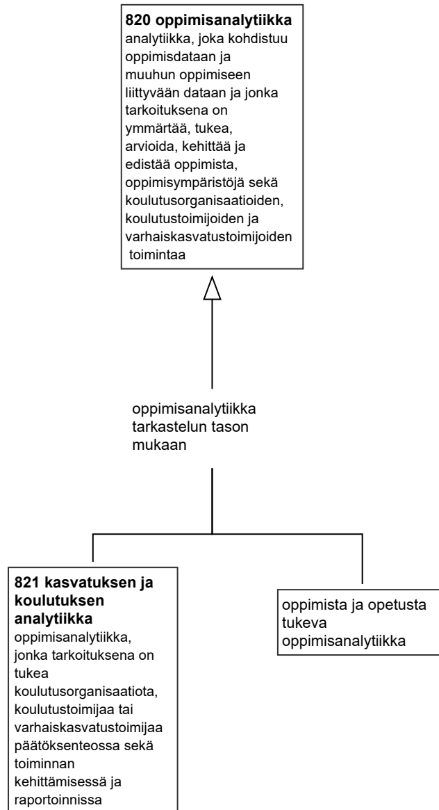
Käsitekaavio 94. Oppimisanalytiikka.
