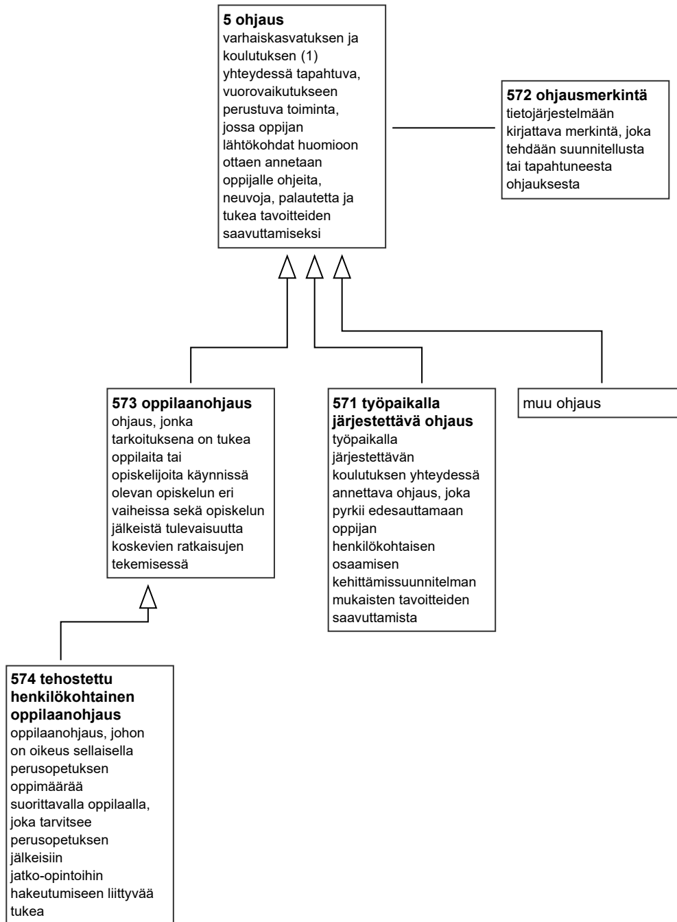
Käsitekaavio 66. Ohjaukäsisteit.
