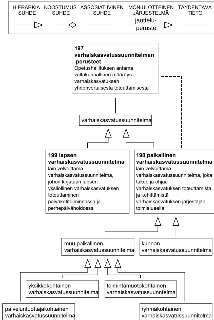
Käsitekaavio 19. Varhaiskasvatussuunnitelmat.
