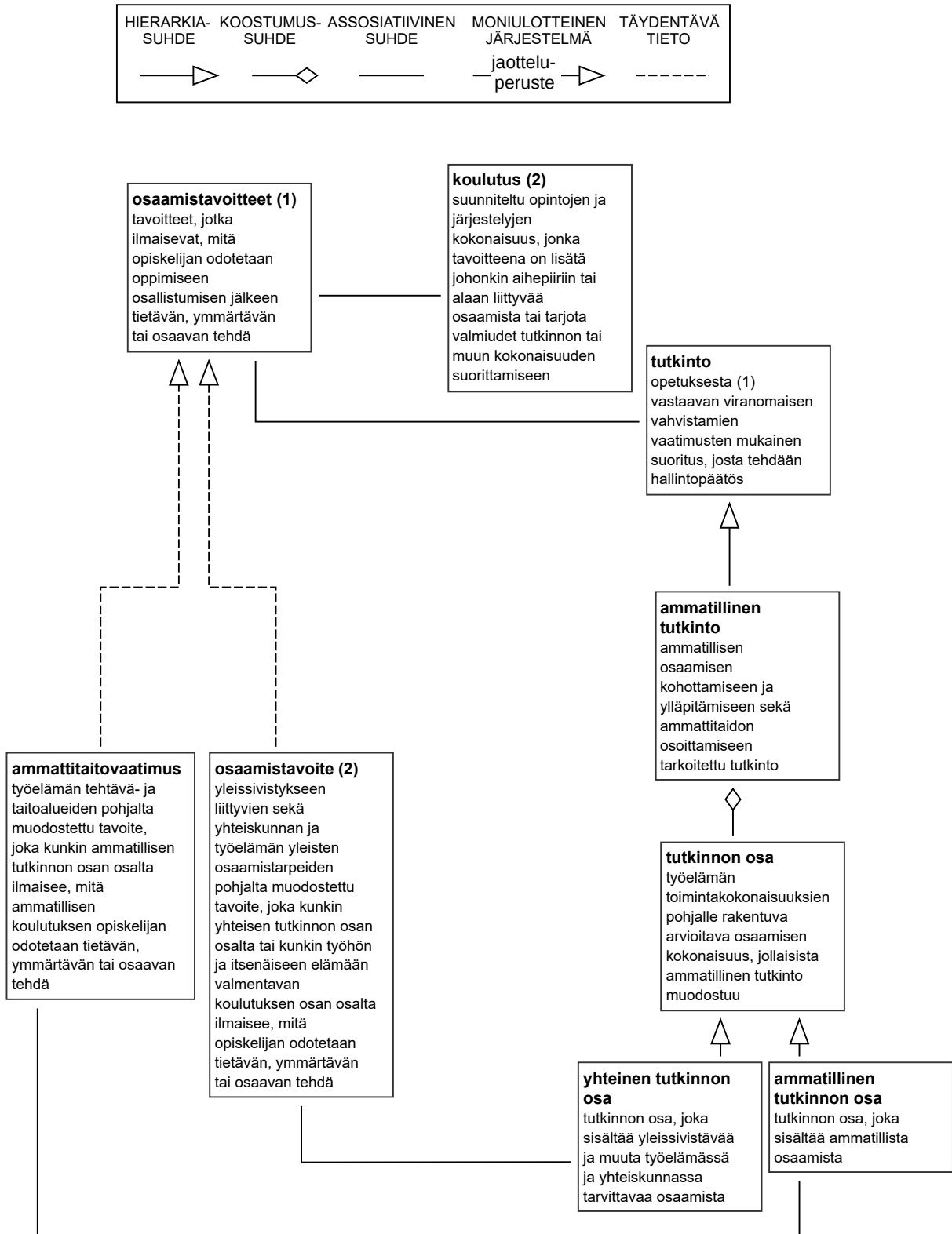
Käsittekaavio 31. Osaamistavoitteet.
