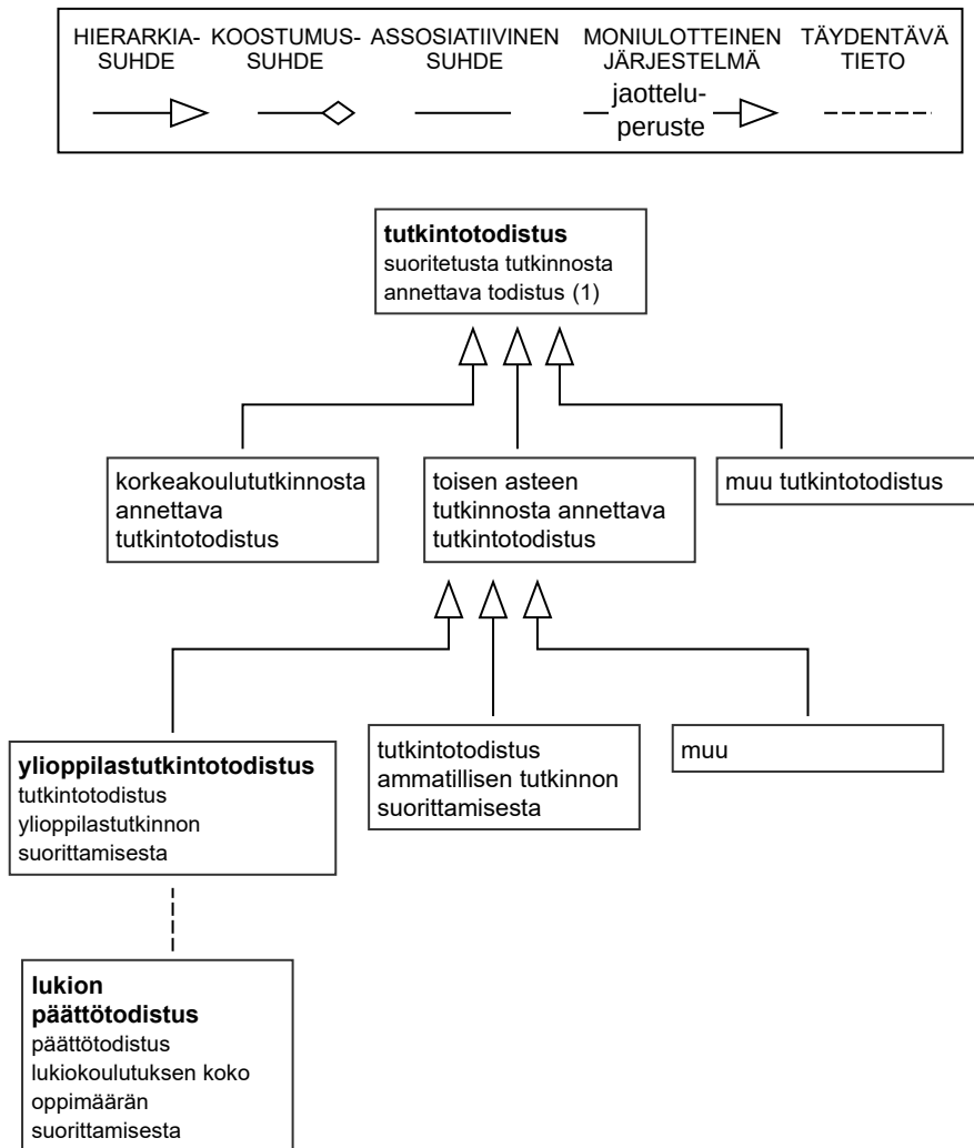
Käsittekaavio 77. Tutkintotodistus.
