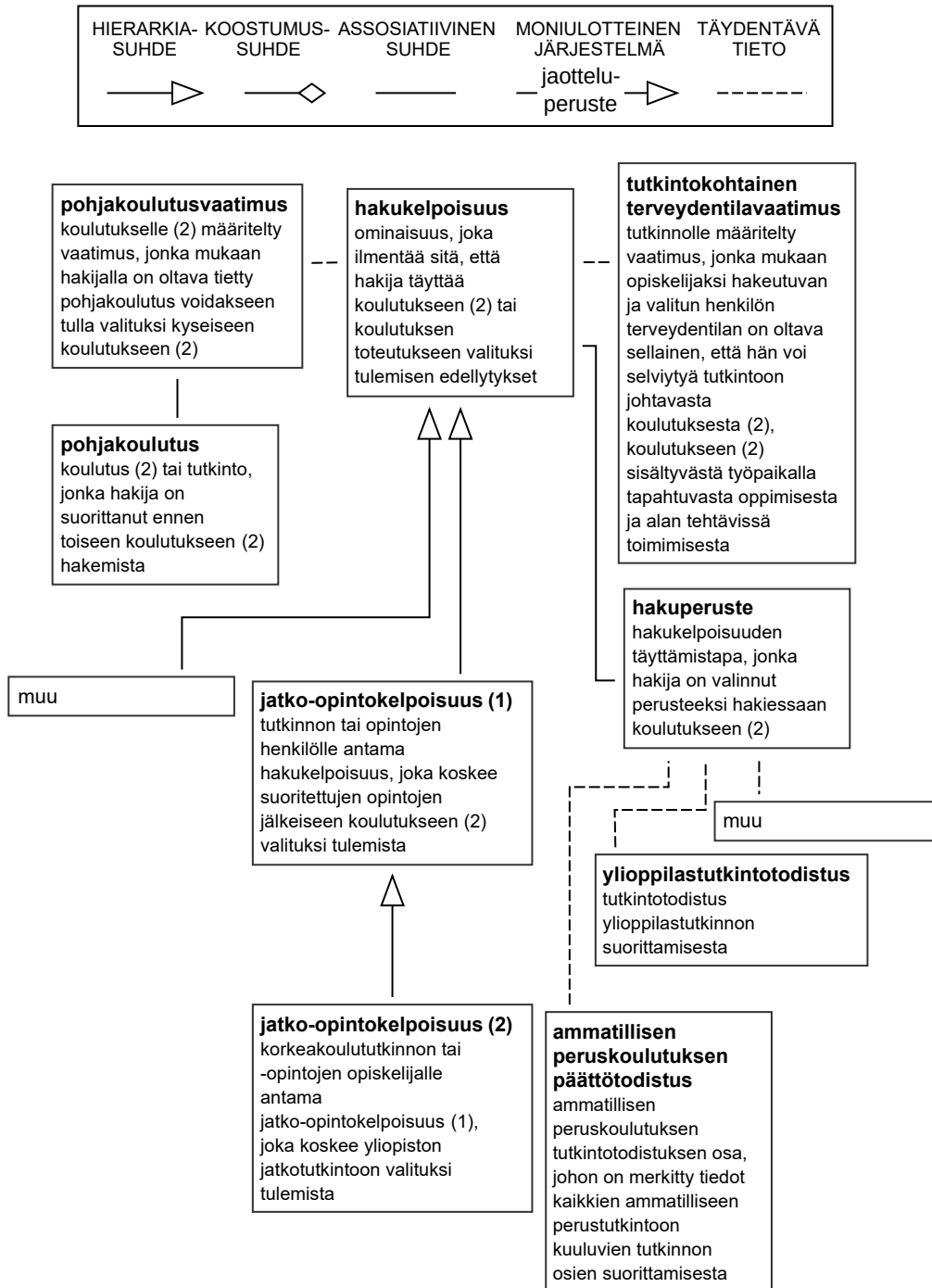
Käsittekaavio 38. Hakukelpoisuus.
