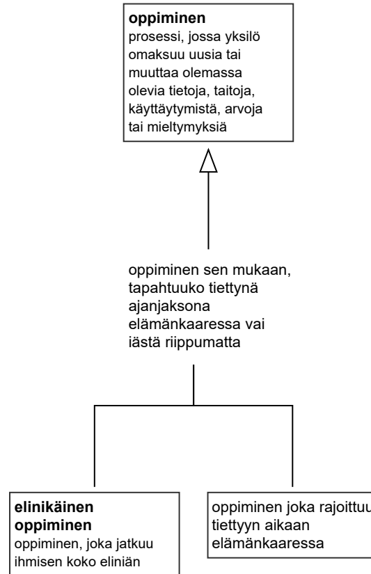
Käsitekaavio 3. Oppiminen.
