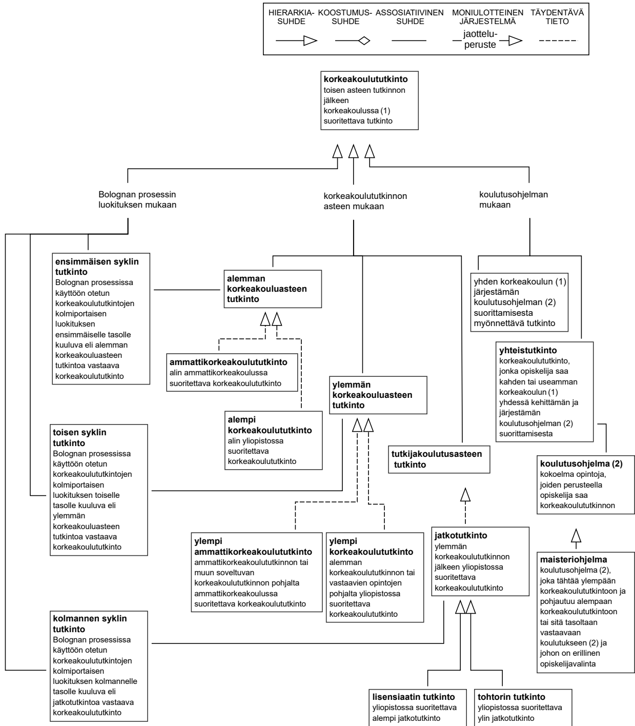
Käsitekaavio 80. Korkeakoulututkinto.
