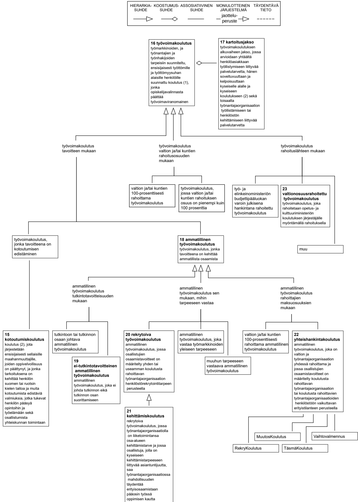
Käsitejärjestelmäkaavio 6. Työvoimakoulutus.
