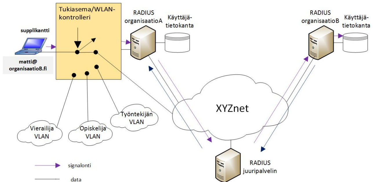
Kuva 5. Autentikointi eduroamissa 802.1x-tekniikkaa soveltaen. Autentikointipyyntö lähetetään RADIUS-hierarkiassa käyttäjän kotiorganisaatioon, jossa käyttäjätunnus ja salasana verrataan tietokantaan tallennettuihin tietoihin.
