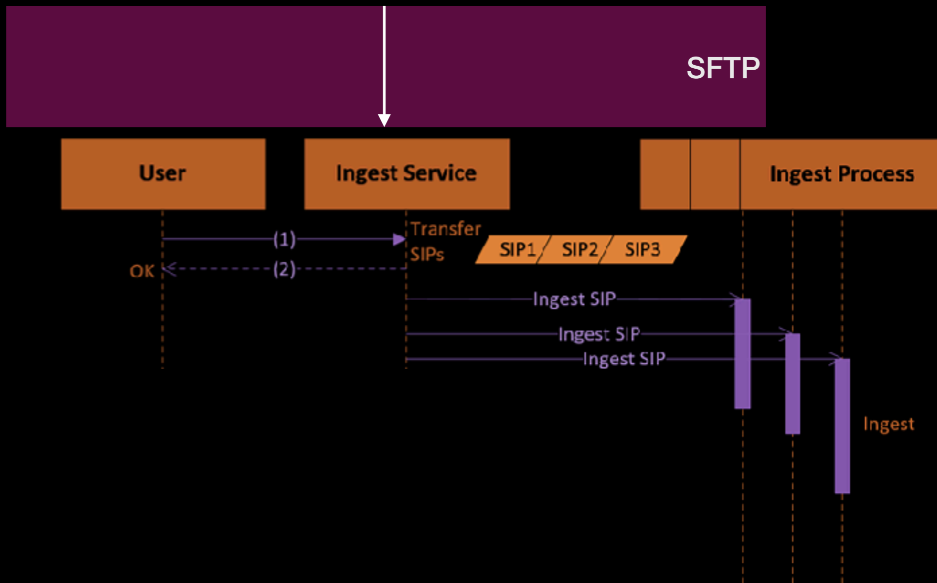
Kuva 1: Aineiston siirtäminen PAS-palveluun ja tarkastusraportin hakeminen.
