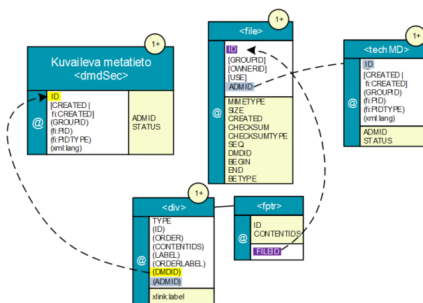
Kuva 7: Attribuuttilinkitykset (esimerkki)
