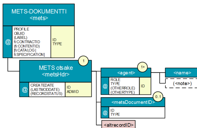
Kuva 3: Osa METS-profiilista
